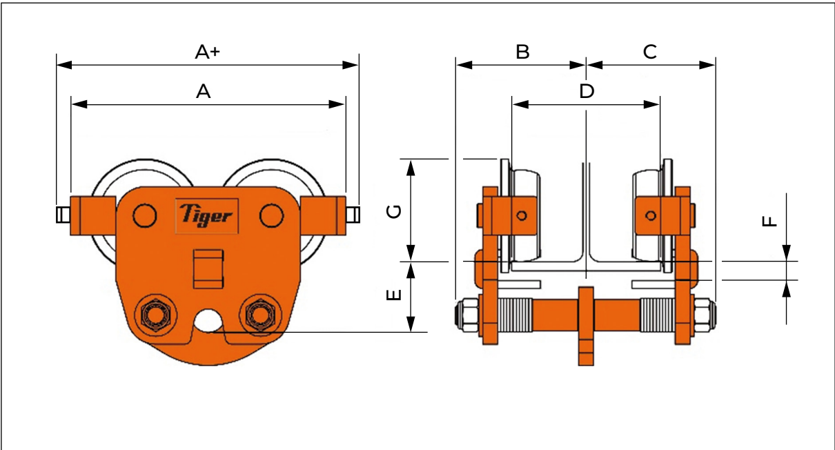
Rollfahrwerk TPT (Zwei Verbindungsbolzen)
