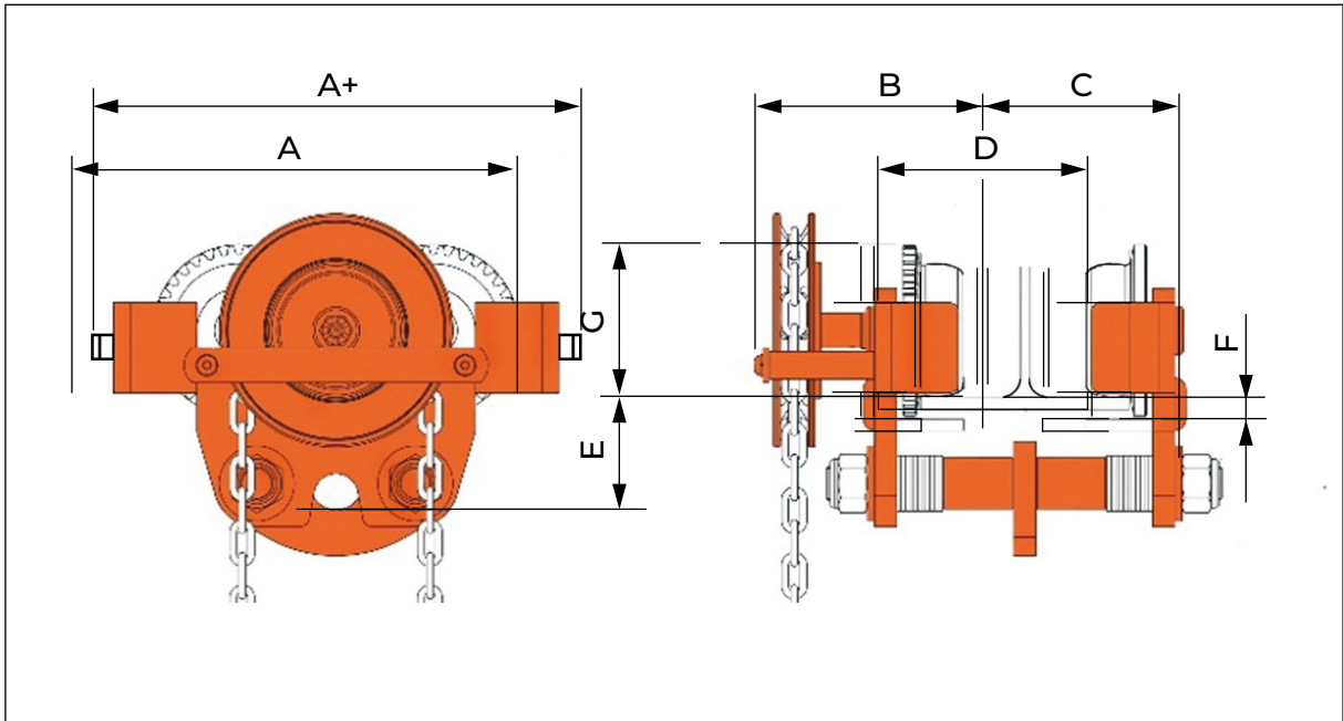
Haspelfahrwerk TGT (Zwei Verbindungsbolzen) 3,0t - 15,0t
