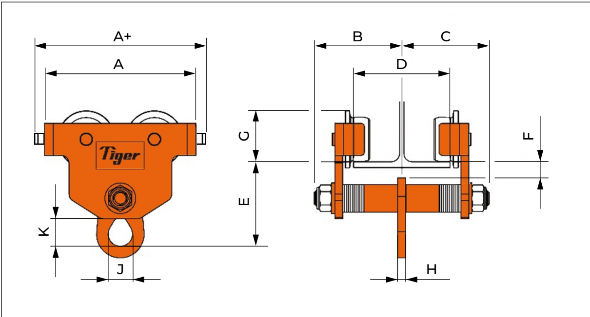
Rollfahrwerk TPS (Ein Verbindungsbolzen)
