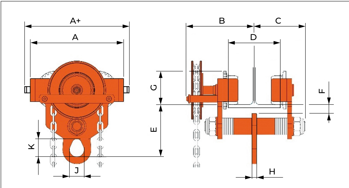
Haspelfahrwerk TGS (Ein Verbindungsbolzen)
