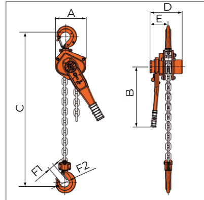
PLH-0320 / 3,0 / 3,2t
