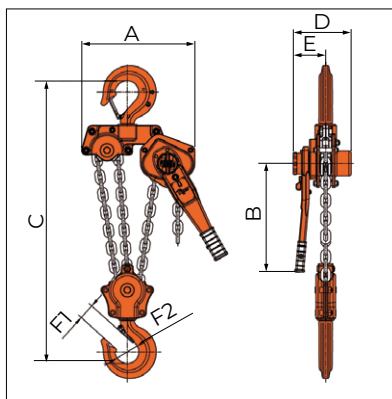
PLH-0630 / 8, t
