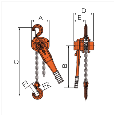
PLH-0160 / 1,5 / 1,6t
