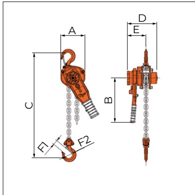
PLH-0080 / 0,8t
